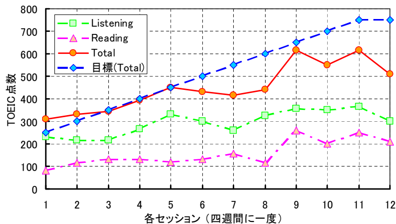
図2 TOEIC スコア
